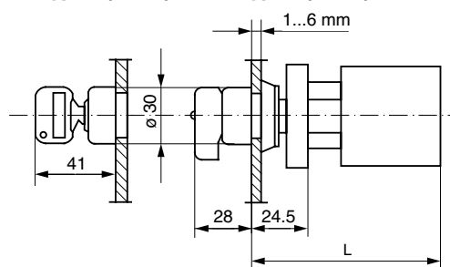
Type D (RC-40)
